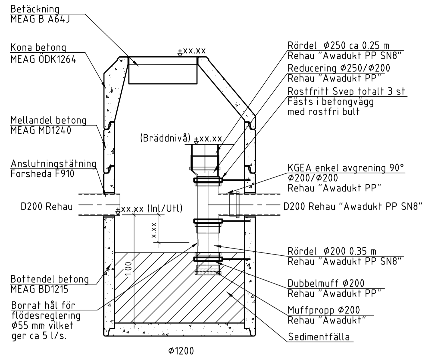
Regleringsbrunn Skala 1:20
